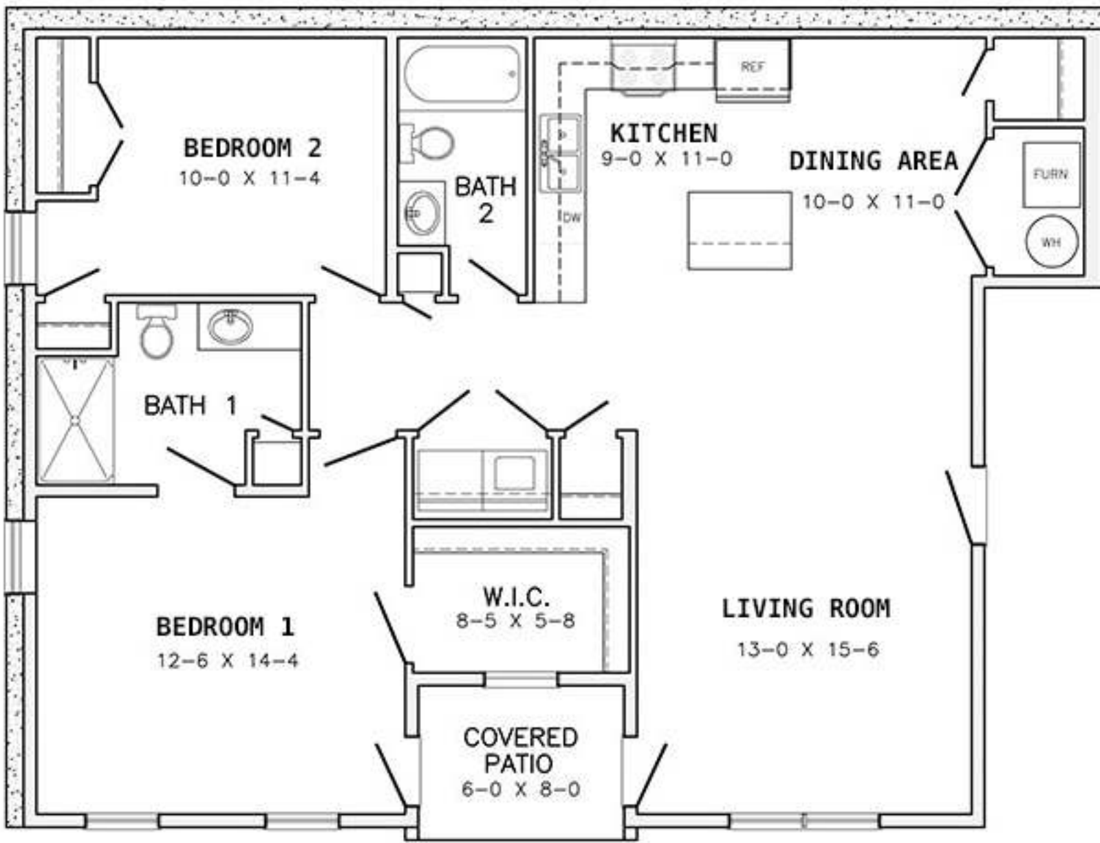
2 BEDRM./ 2 BATH FLOOR PLAN 1183 S.F.
